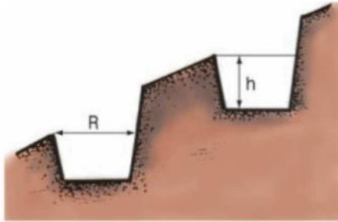
Hình 34. Đào hố trên đất dốc R : Chiều rộng của hố. h : Chiều sâu của hố
